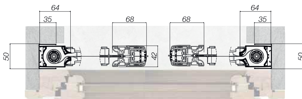
FLASH MAXI INCASSO 2 ANTE
