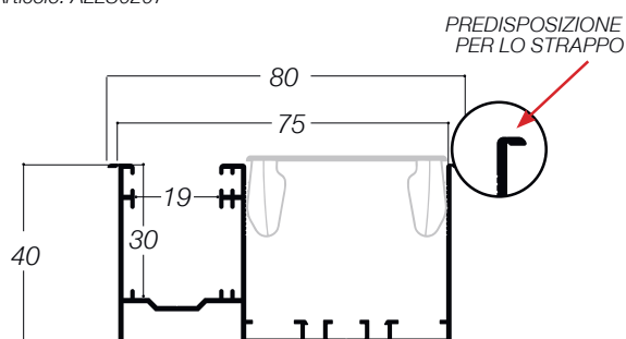
PROFILO INCASSATA 45-80 TAPPARELLA 758 gr/ml - costo stabilito dall'andamento del mercato Articolo: ALLU0207
