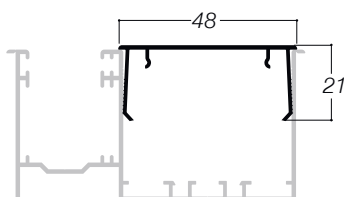
CARTER IN ALLUMINIO Articolo: ALLU0231
