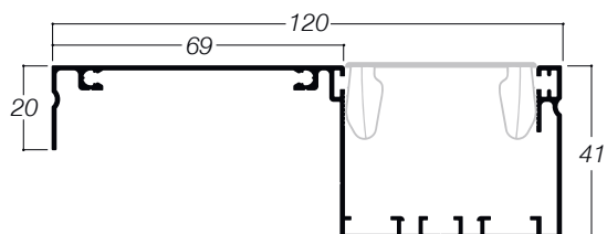
PROFILO INCASSATA 45 PERSIANA 868 gr/ml - costo stabilito dall'andamento del mercato Articolo: ALLU0256
