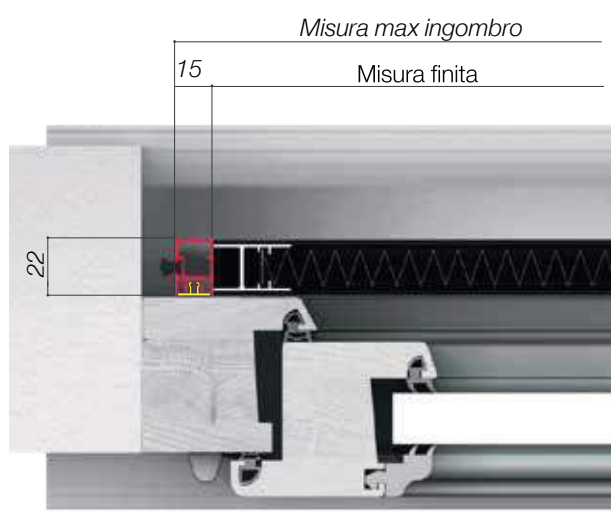
FISSAGGIO CON CLIP SEZ. ORIZZONTALE
