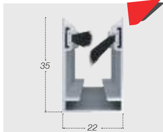
Spazzolino antivento
