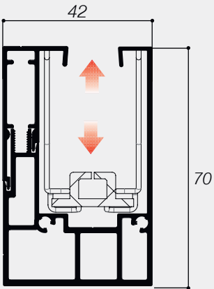
GUIDA MAGGIORATA 70 mm
