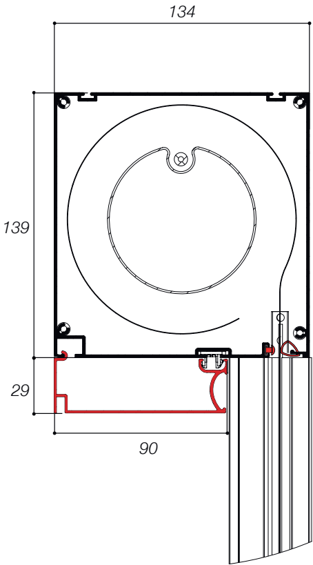
CASSONETTO 130 mm
