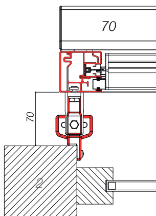
SUPPORTO FISSO AD ANGOLO
