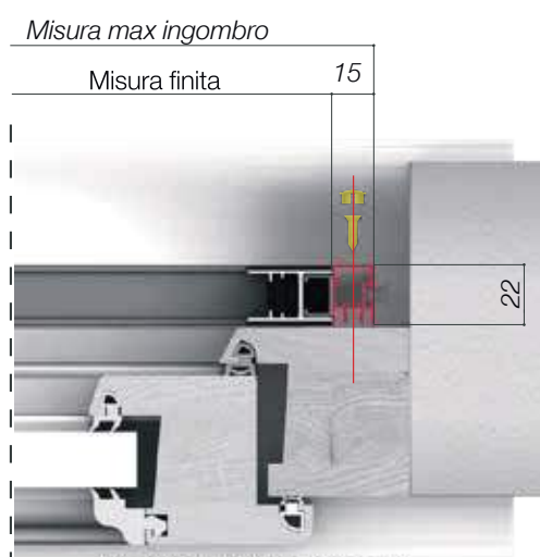
FISSAGGIO CON VITE SEZ. ORIZZONTALE
