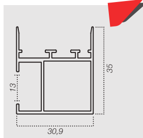
Profilo di chiusura alto
