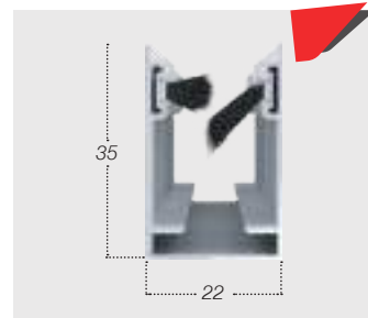
Spazzolino antivento
