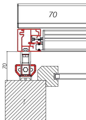
SUPPORTO FISSO PIANO
