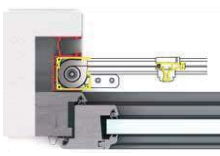
UNIKA 45 LATERALE Articolo: ZANL026
