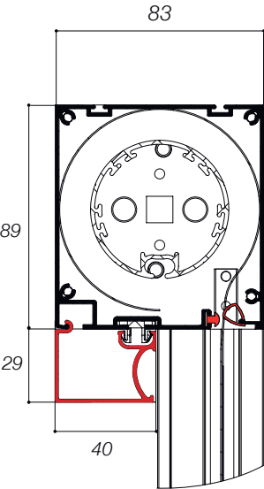
CASSONETTO 80 mm
