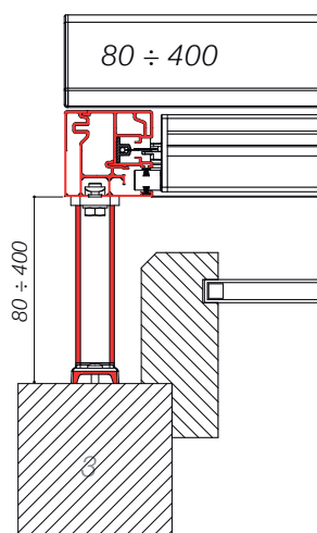
SUPPORTO VARIABILE PIANO
