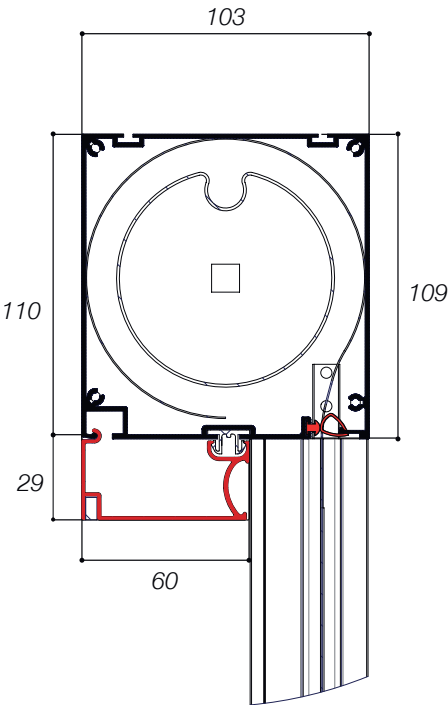
CASSONETTO 100 mm
