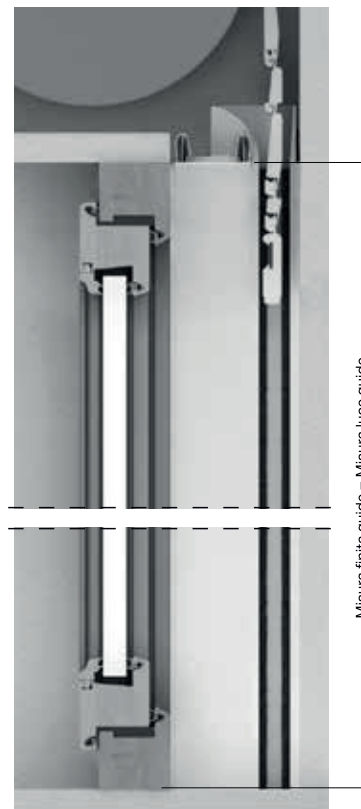
PROFILI INCASSATA 45-80 TAPPARELLA
