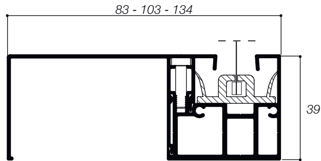
GUIDA INCASSO
