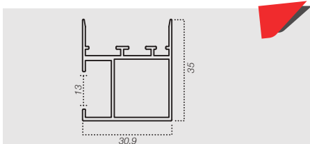
Profilo di chiusura alto
