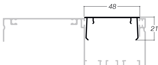
CARTER IN ALLUMINIO Articolo: ALLU0231
