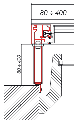
SUPPORTO VARIABILE AD ANGOLO
