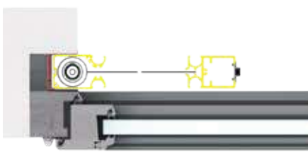
ZERO - FLASH Articolo: ZANL011 Articolo: ZANL012
