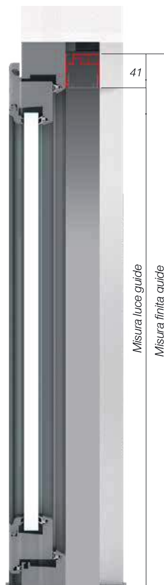
SEZ. VERTICALE
