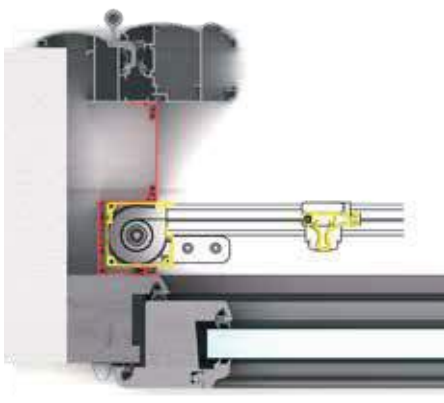
UNIKA 45 LATERALE Articolo: ZANL026
