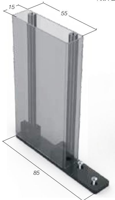
TUBOLARE 55 x 15 Art. ALLU0595
