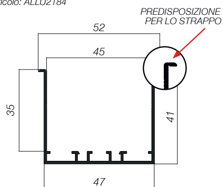
PROFILO INCASSATA 45 Articolo: ALLU2184
