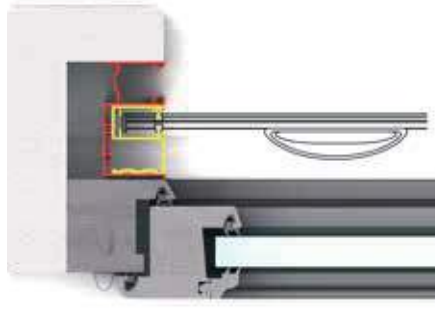
UNIKA 45 VERTICALE Articolo: ZANV025
